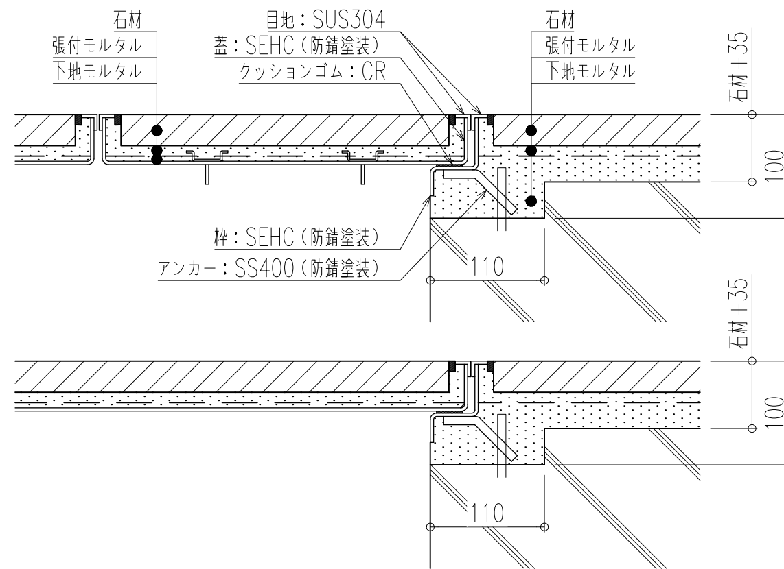
施工参考拡大図
